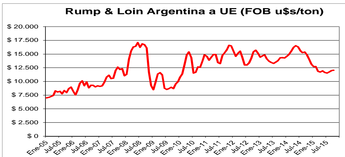
Gráfico n° 7: Precio promedio de exportación y volumen exportado del Rump & Loin Argentina a la Unión Europea (incluye operaciones dentro y fuera de cuota)
